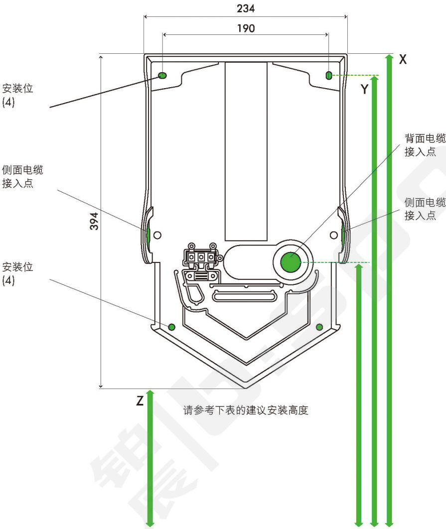
背视图
